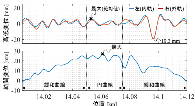
図 4 高低変位と軌間変位の検出データ例
