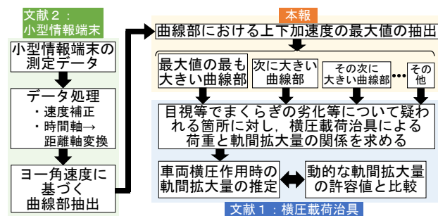
図7 軌間拡大リスクの評価手順
