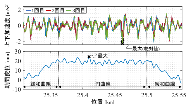
図 5 軌間変位の検出データと列車動揺データの例
